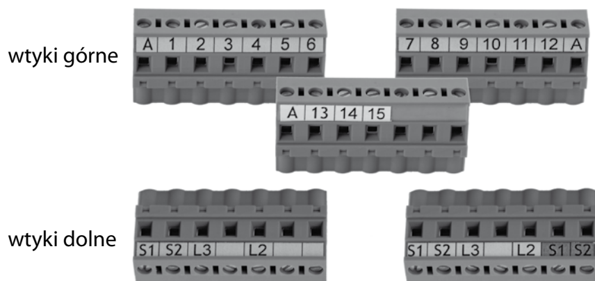
Rys. 4. Rysunek wtyków do regulatora z rozmieszczeniem i oznaczeniem zacisków aktywnych
