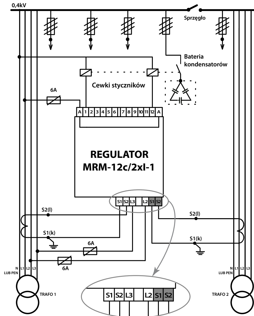
Rys.7. Schemat podłączenia regulatora MRM - 12c/2xI - 1 (podwójne wejście prądowe)
